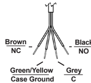
Cable
